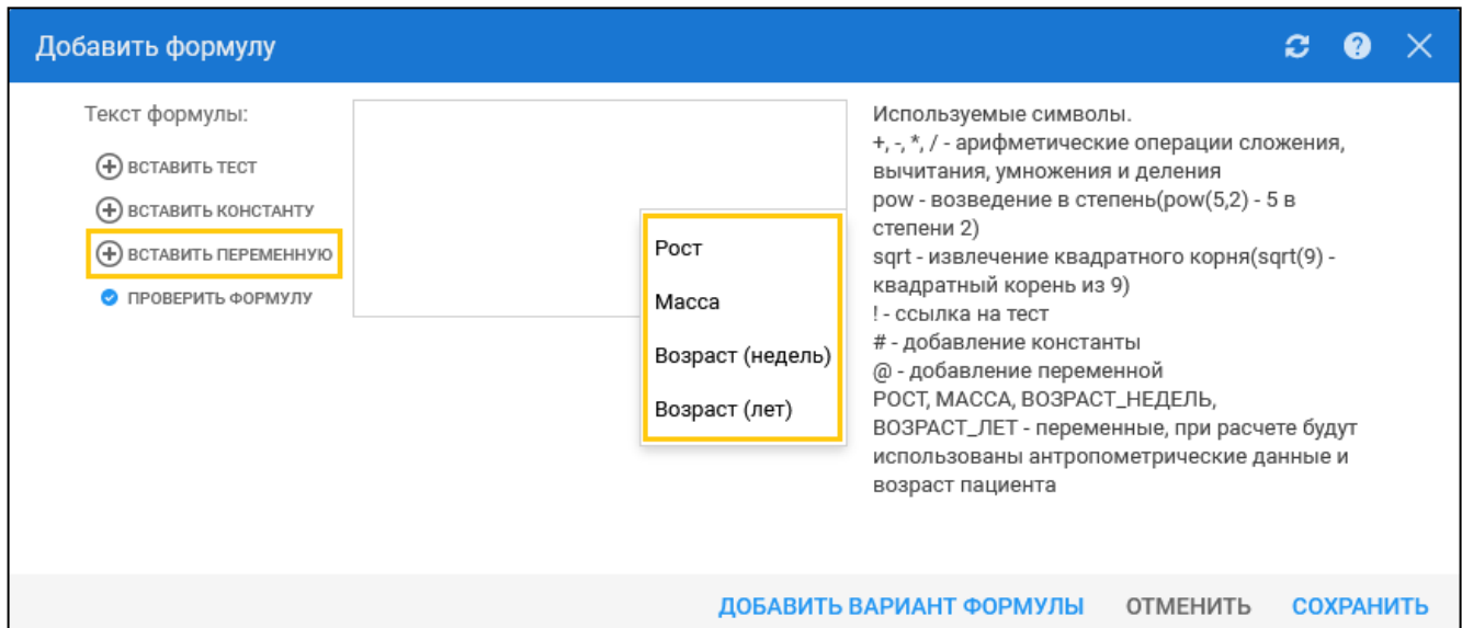
Рисунок 201 – Добавление переменной
